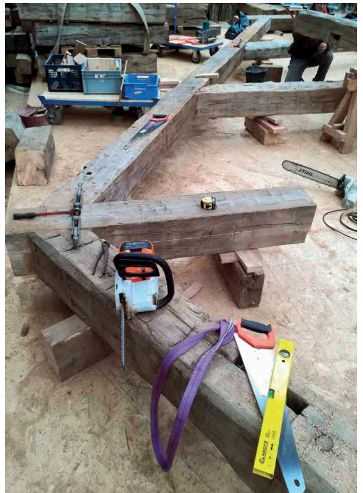
Pré-montage / Pre-assembly
